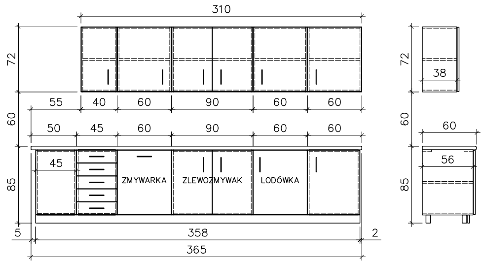
Rys. Z-2
