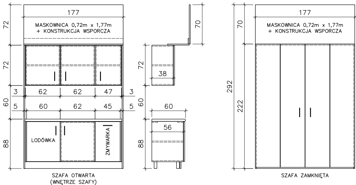
Rys. Z-3
